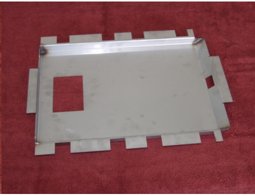
Fire Pan
